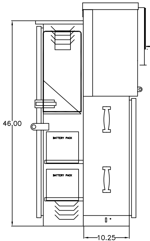
LEFT SIDE
